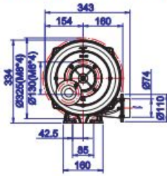
HTB75-032 2-stage
