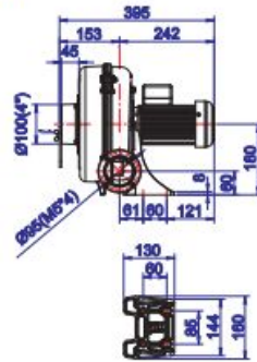
HTB75-032 2-stage
