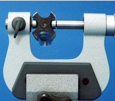
测量丝锥根部尺寸
