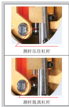
杠杆结构
