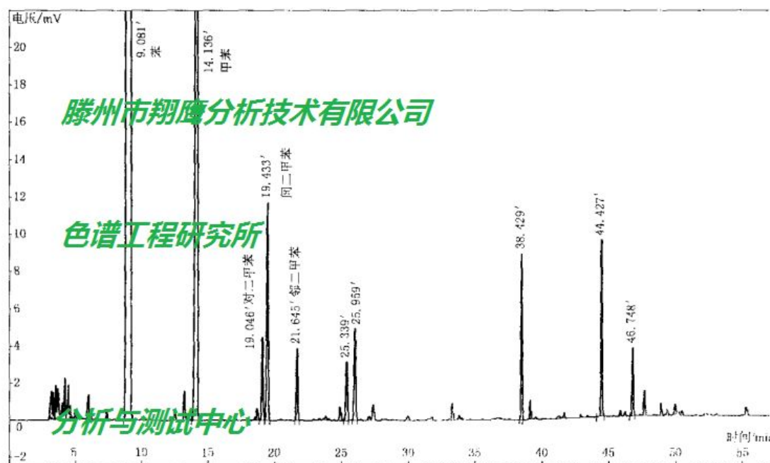
粗苯中组分的典型色谱图
