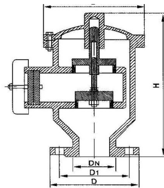
结构示意图
