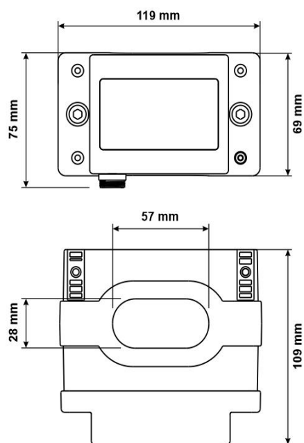
分体式传感器尺寸图
