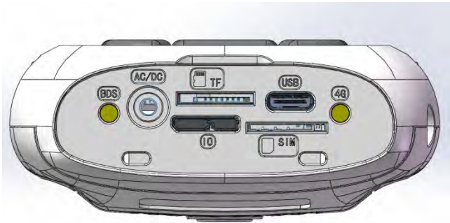
图 4-1-4 底部接口
