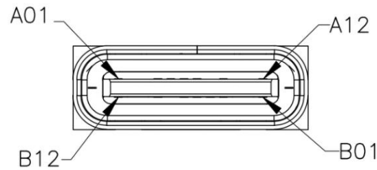
图 4-1-7 USB 串口引脚
