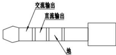
图 4-1-5 立体声插头引脚
