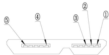
图 4-1-8 IO 串口引脚
