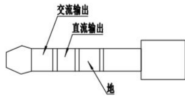
图 4-5 立体声插头引脚
