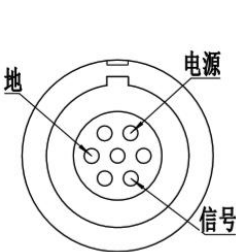
图 4-3 插座引脚
