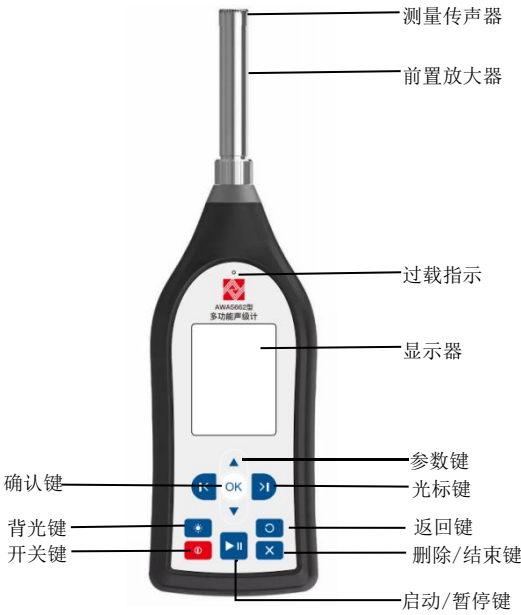
图 4-1 仪器正面
