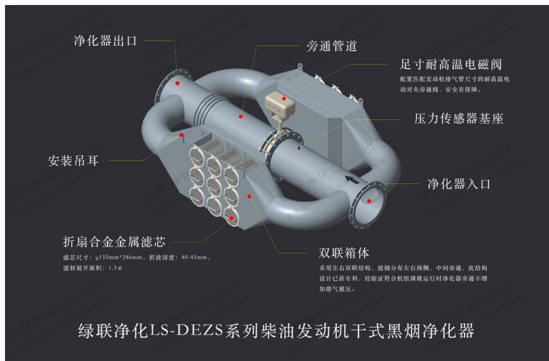
绿联净化 LS-DEZS 系列柴油发动机干式黑烟净化器
